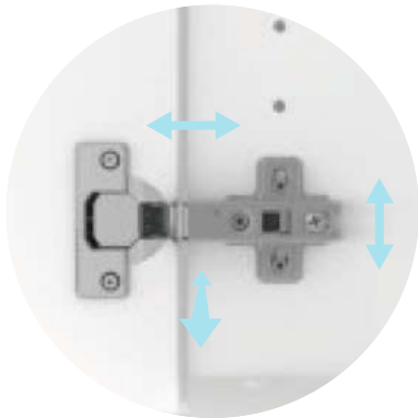
anta con cerniera regolabile montata door with levelling hinge porte avec charnière réglable montée Tür mit montiertem einstellbarem Scharnier deur met gemonteerd, verstelbaar scharnier puerta con bisagra regulable montada
